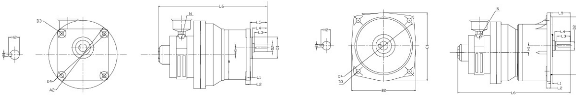
M420FX-M408/M420FX-M151 dimensions
